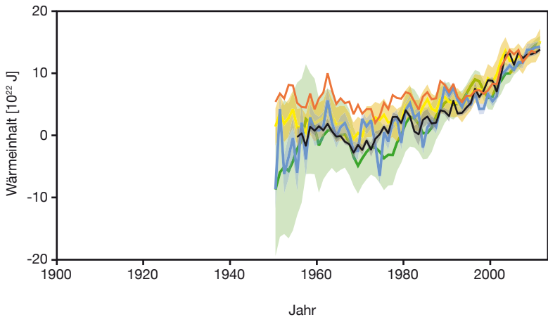
a: Änderung des global gemittelten Wärmehalts der oberen Ozeanschichten
