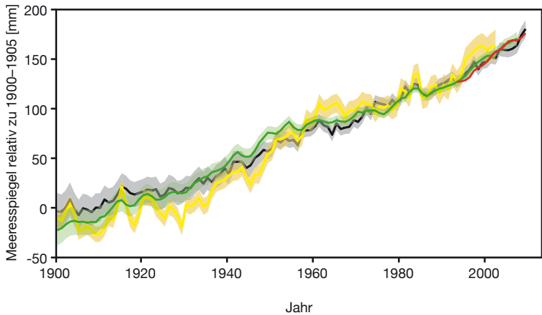
b: Global gemittelter Meeresspiegelanstieg
